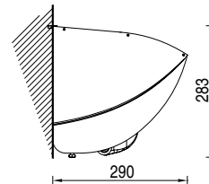
Installazione con tettuccio. Installation with hood
