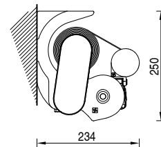
Installazione a parete con staffa parete/soffitto. Wall installation with wall/ceiling bracket
