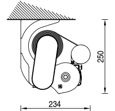
Installazione a soffitto con staffa parete/soffitto. Ceiling installation with wall/ceiling bracket
