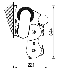
Installazione con bracci incrociati. Crossed arms installation
