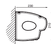
Montering med baldakin Installation with a hood
